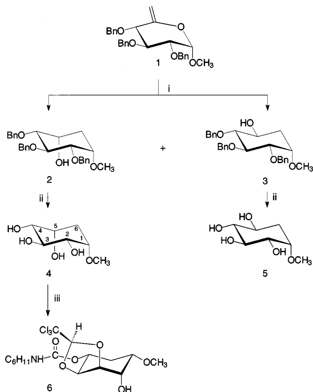
Scheme 2. i: i\text{Bu}_3\text{Al} (toluene); [12] ii: \text{H}_2 , Pd/C (MeOH/EtOAc); iii: DCC, chloral
